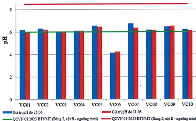
Hình 2: Biểu đồ giá trị pH tại các vị trí lấy mẫu ngày 24-26/06
