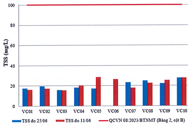
Hình 4: Biểu đồ giá trị TSS tại các vị trí lấy mẫu ngày 24-26/06
