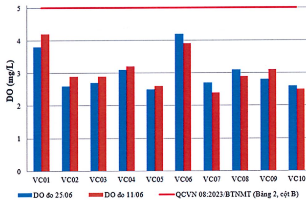
Hình 5: Biểu đồ giá trị DO tại các vị trí lấy mẫu ngày 24-26/06
