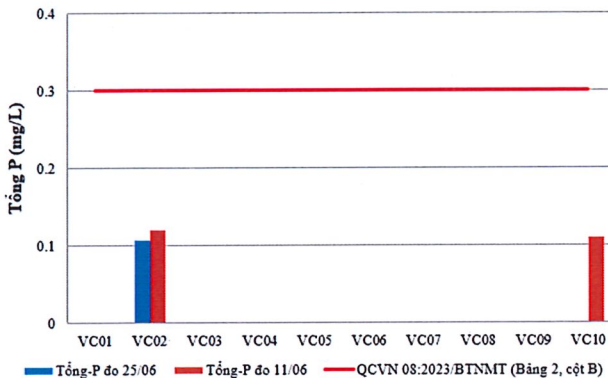
Hình 8: Biểu đồ giá trị tổng P tại các vị trí lấy mẫu ngày 24-26/06
