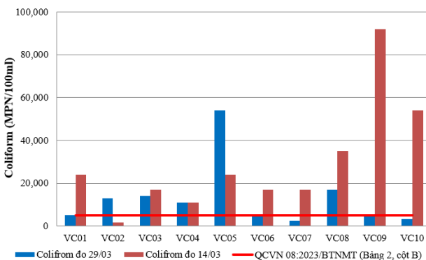
Hình 9: Biểu đồ giá trị Coliform tại các vị trí lấy mẫu ngày 28-30/03
