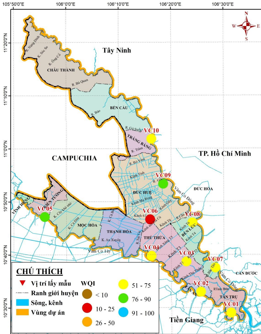
Hình 10: Biểu thị chỉ số WQI tại các vị trí lấy mẫu ngày 28-30/03/2025
