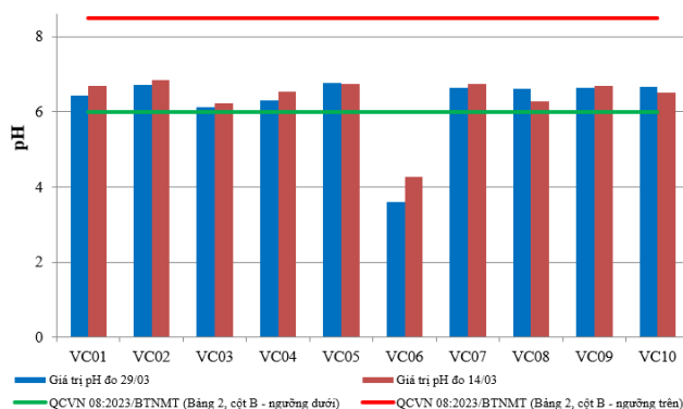
Hình 2: Biểu đồ giá trị pH tại các vị trí lấy mẫu ngày 28-30/03
