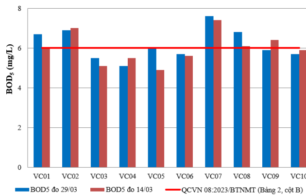
Hình 6: Biểu đồ giá trị BOD 5 tại các vị trí lấy mẫu ngày 28-30/03
