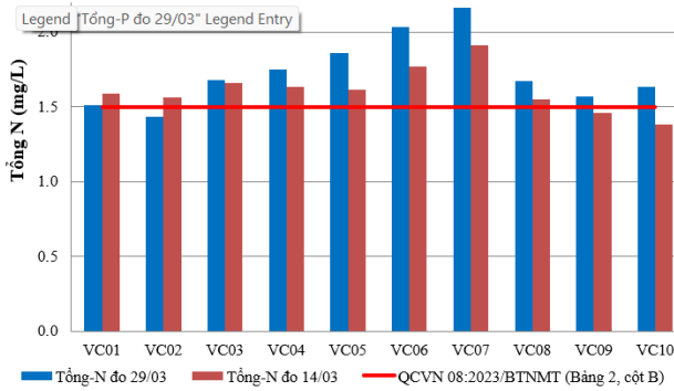
Hình 7: Biểu đồ giá trị tổng N tại các vị trí lấy mẫu ngày 28-30/03
