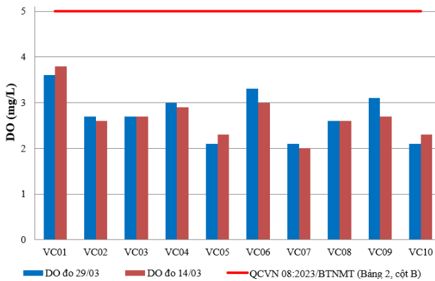
Hình 5: Biểu đồ giá trị DO tại các vị trí lấy mẫu ngày 28-30/03
