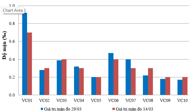
Hình 3: Biểu đồ giá trị mặn tại các vị trí lấy mẫu ngày 28-30/03
