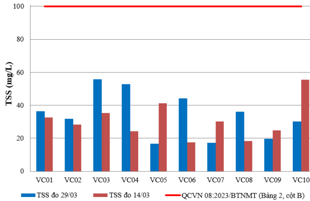
Hình 4: Biểu đồ giá trị TSS tại các vị trí lấy mẫu ngày 28-30/03
