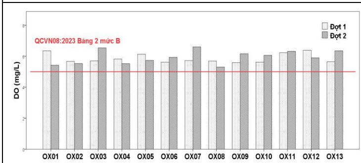
Hình 7. Giá trị DO tại các vị trí quan trắc
