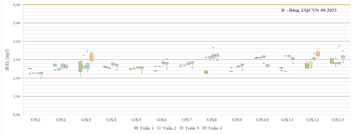
Hình 12. Kết quả dự báo diễn biến BOD 5 trong các tuần tháng 03/2025
