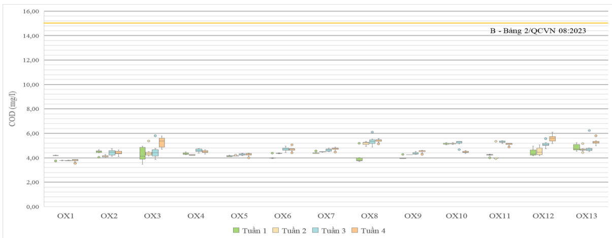
Hình 13. Kết quả dự báo diễn biến COD trong các tuần tháng 03/2025
