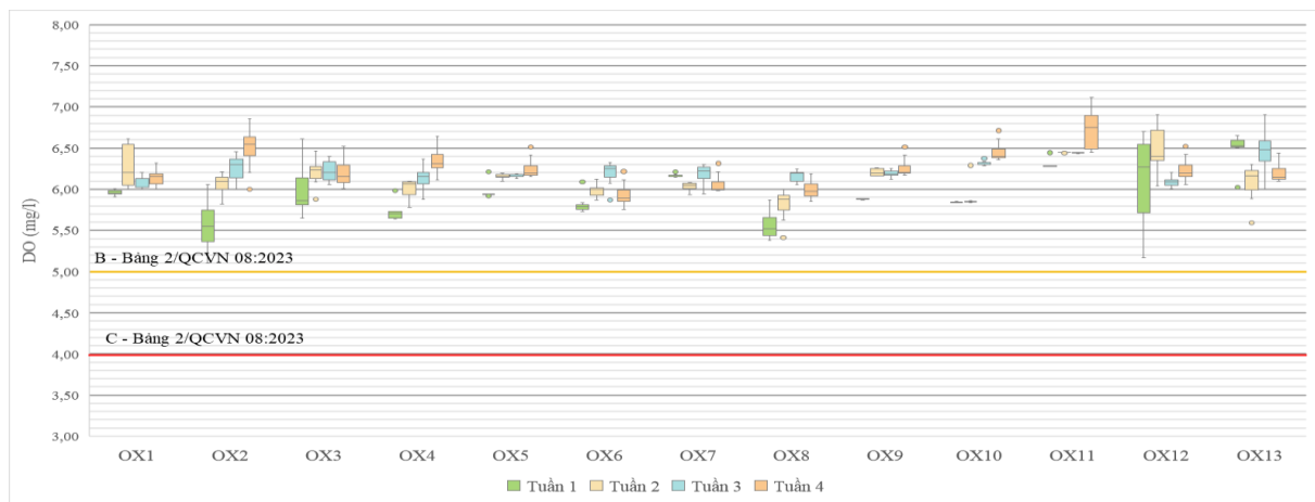
Hình 11. Kết quả dự báo diễn biến DO trong các tuần tháng 03/2025
