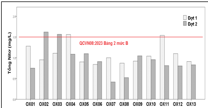
Hình 8. Giá trị TN tại các vị trí quan trắc
