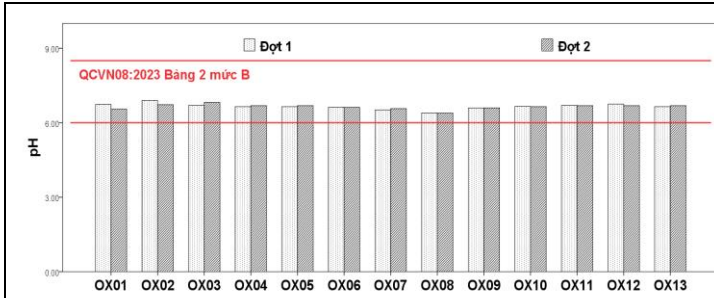
Hình 2. Giá trị pH tại các vị trí quan trắc
