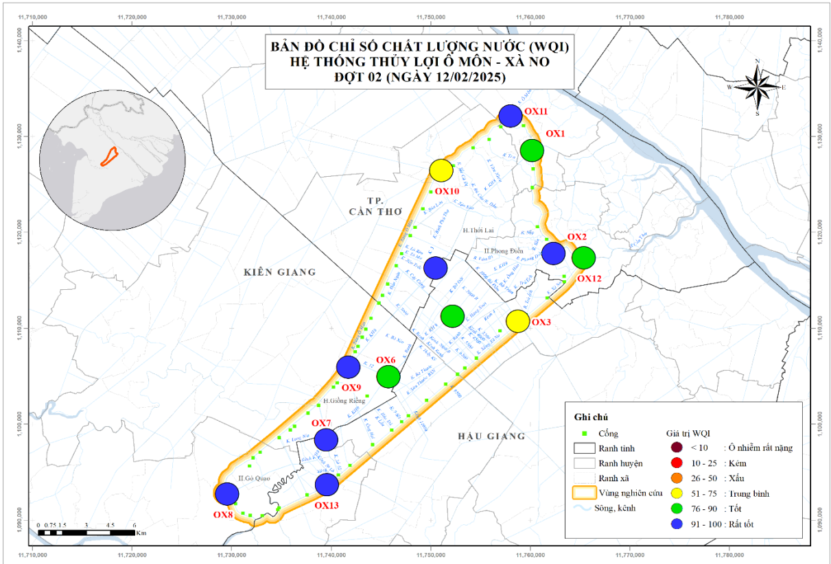
Hình 2. Giá trị WQI chất lượng nước vùng Ô Môn – Xà No đợt 2 – ngày 12/02/2025
