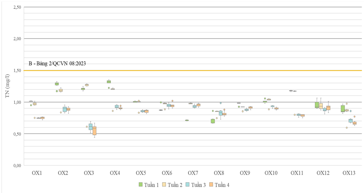
Hình 14. Kết quả dự báo diễn biến TN trong các tuần tháng 03/2025
