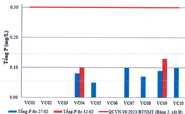
Hình 8: Biểu đồ giá trị tổng P tại các vị trí lấy mẫu ngày 26-28/02
