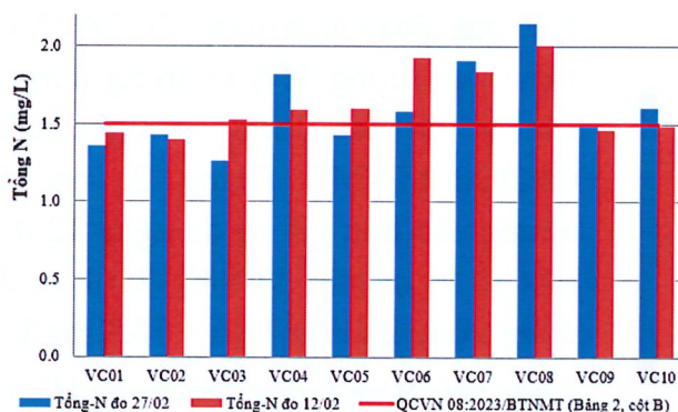
Hình 7: Biểu đồ giá trị tổng N tại các vị trí lấy mẫu ngày 26-28/02
