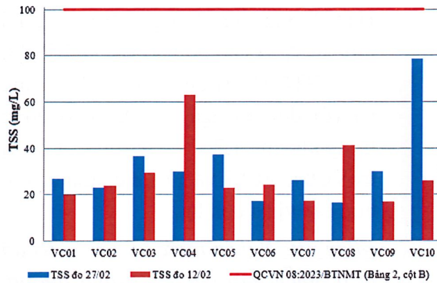
Hình 4: Biểu đồ giá trị TSS tại các vị trí lấy mẫu ngày 26-28/02
