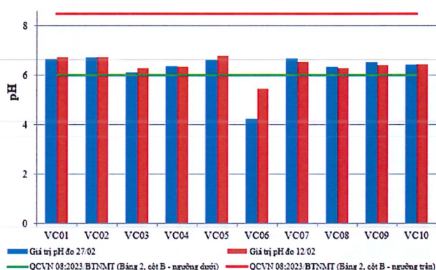
Hình 2: Biểu đồ giá trị pH tại các vị trí lấy mẫu ngày 26-28/02
