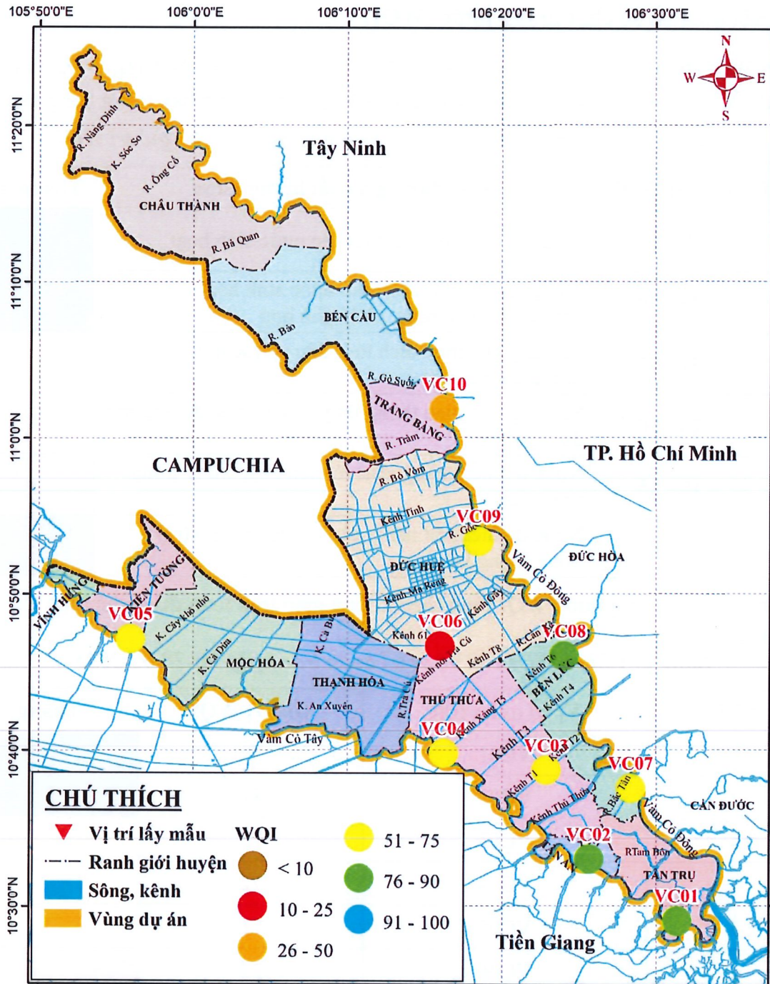
Hình 10: Biểu thị chỉ số WQI tại các vị trí lấy mẫu ngày 26-28/02/2025
