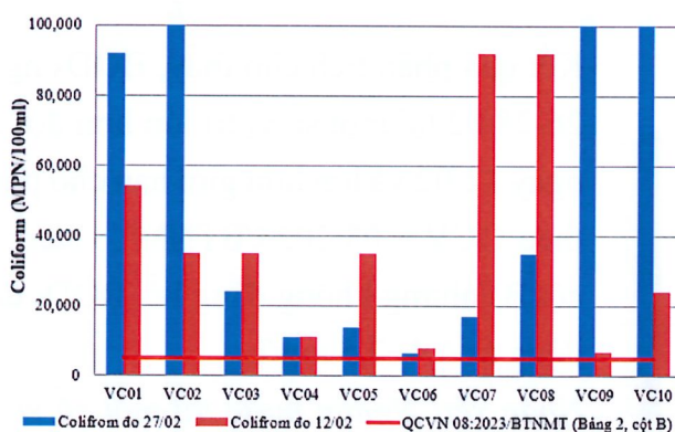
Hình 9: Biểu đồ giá trị Coliform tại các vị trí lấy mẫu ngày 26-28/02
