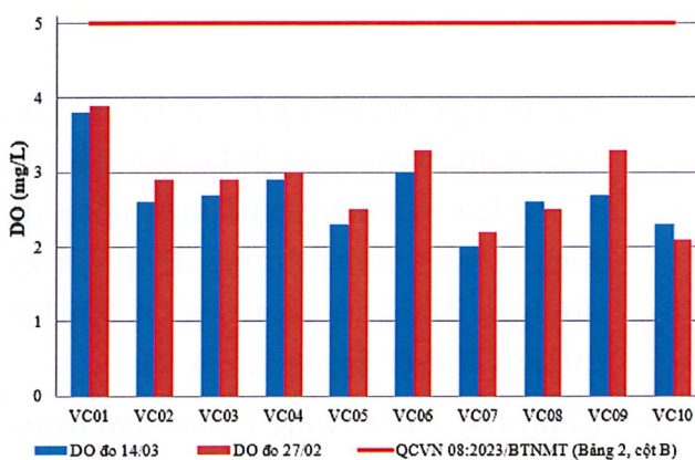
Hình 5: Biểu đồ giá trị DO tại các vị trí lấy mẫu ngày 13-15/03
