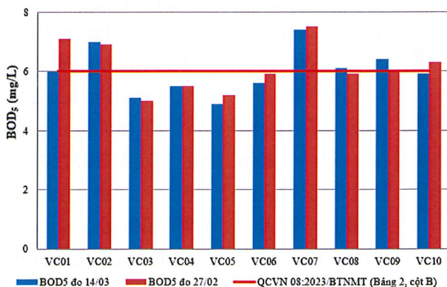
Hình 6: Biểu đồ giá trị BOD 5 tại các vị trí lấy mẫu ngày 13-15/03
