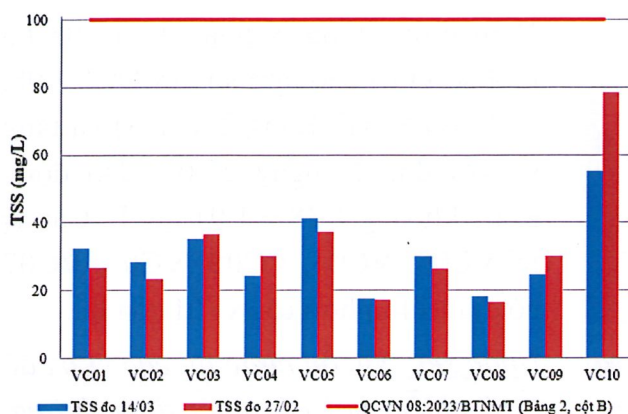
Hình 4: Biểu đồ giá trị TSS tại các vị trí lấy mẫu ngày 13-15/03
