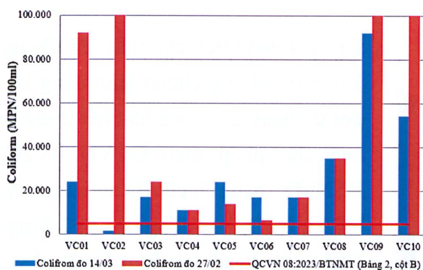
Hình 9: Biểu đồ giá trị Coliform tại các vị trí lấy mẫu ngày 13-15/03
