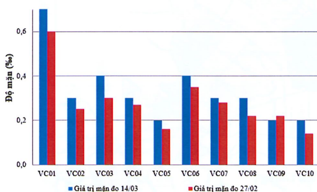
Hình 3: Biểu đồ giá trị mặn tại các vị trí lấy mẫu ngày 13-15/03
