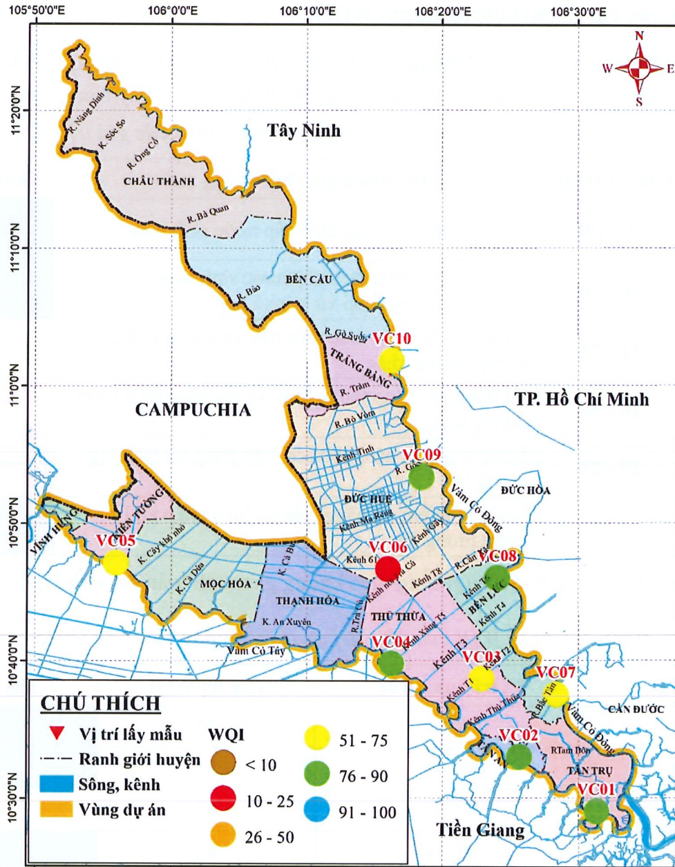
Hình 10: Biểu thị chỉ số WQI tại các vị trí lấy mẫu ngày 13-15/03/2025
