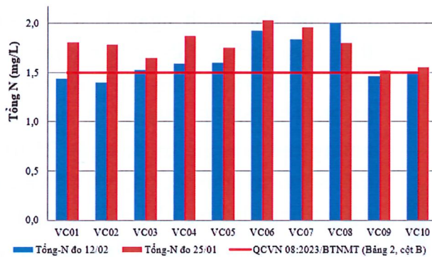
Hình 7: Biểu đồ giá trị tổng N tại các vị trí lấy mẫu ngày 11-13/02
