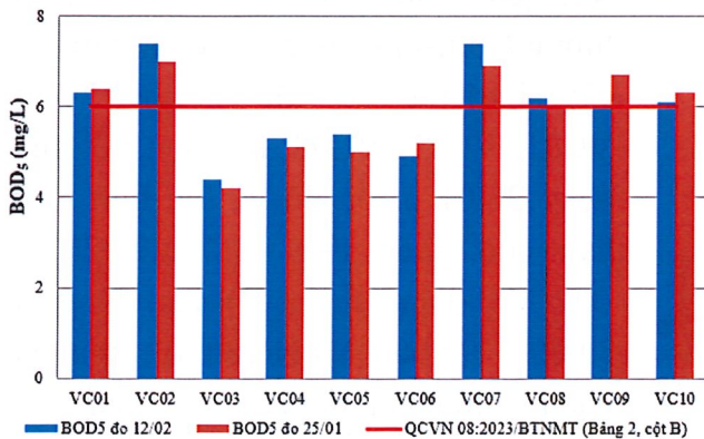
Hình 6: Biểu đồ giá trị BOD 5 tại các vị trí lấy mẫu ngày 11-13/02
