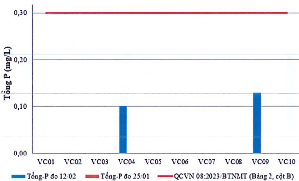
Hình 8: Biểu đồ giá trị tổng P tại các vị trí lấy mẫu ngày 11-13/02
