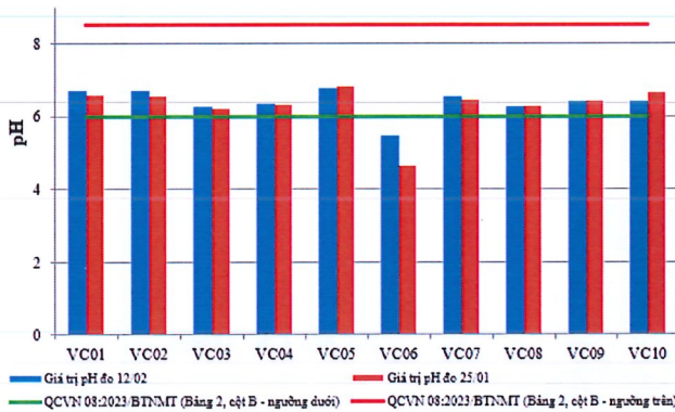
Hình 2: Biểu đồ giá trị pH tại các vị trí lấy mẫu ngày 11-13/02
