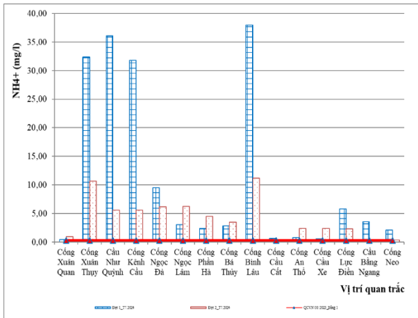
Hình 2.9. Diễn biến hàm lượng NH_4^+ các đợt quan trắc trong tháng 7/2024
