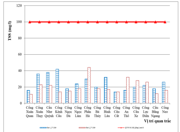
Hình 2.5. Diễn biến hàm lượng TSS các đợt quan trắc trong tháng 7/2024
