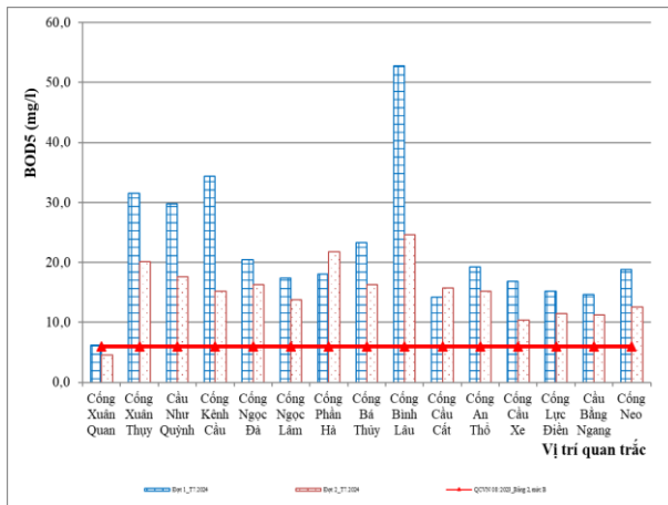
Hình 2.6. Diễn biến hàm lượng BOD 5 các đợt quan trắc trong tháng 7/2024
