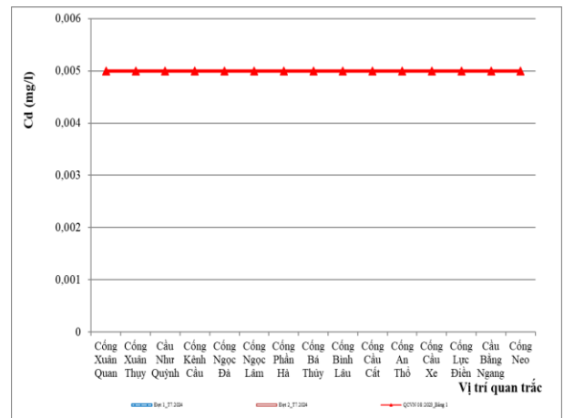
Hình 2.12. Diễn biến hàm lượng Cd các đợt quan trắc trong tháng 7/2024
