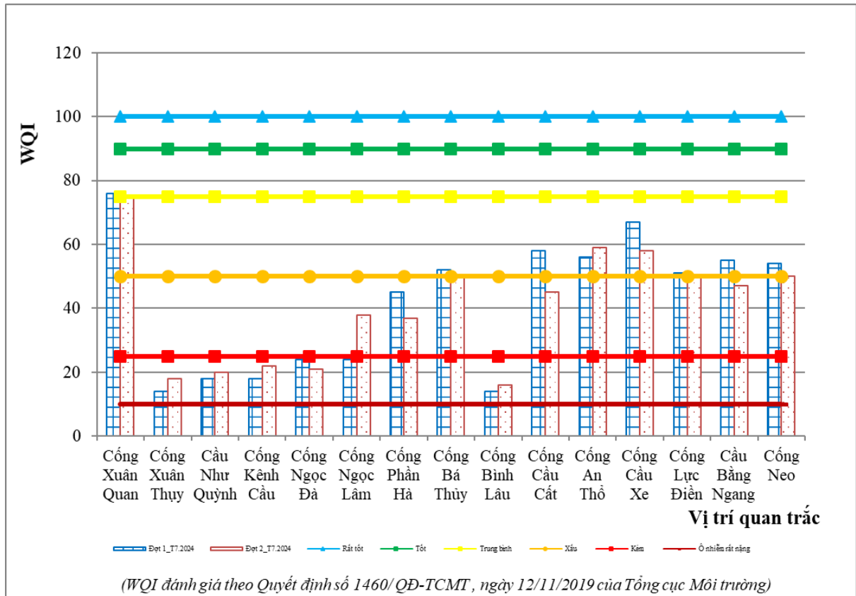
Hình 2.1. Diễn biến chỉ số WQI các đợt quan trắc trong tháng 7/2024
