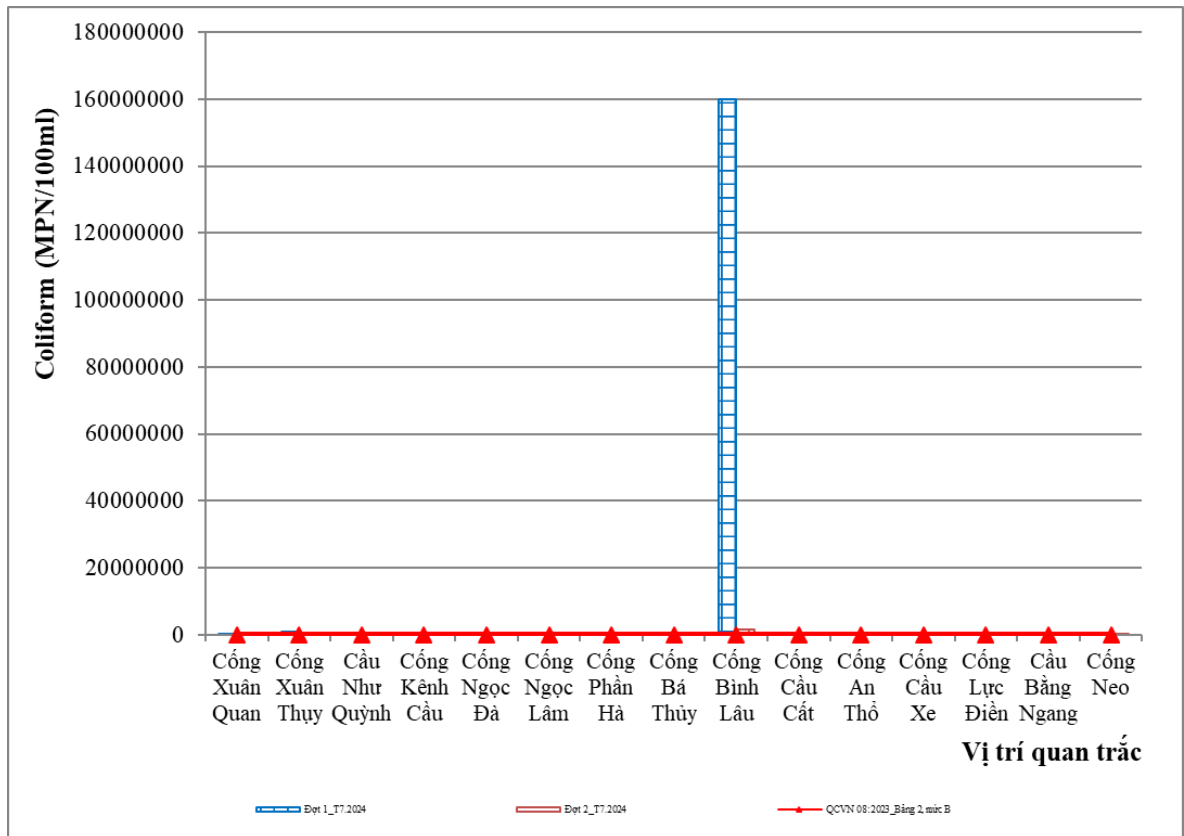
Hình 2.8. Diễn biến hàm lượng Coliform các đợt quan trắc trong tháng 7/2024
