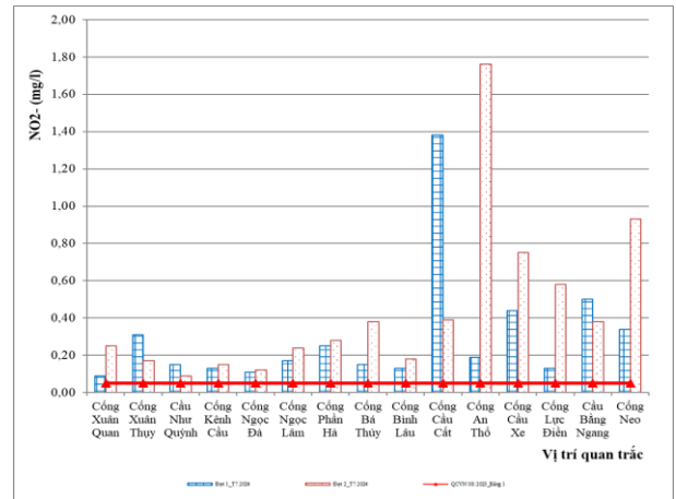
Hình 2.10. Diễn biến hàm lượng NO_2^- các đợt quan trắc trong tháng 7/2024
