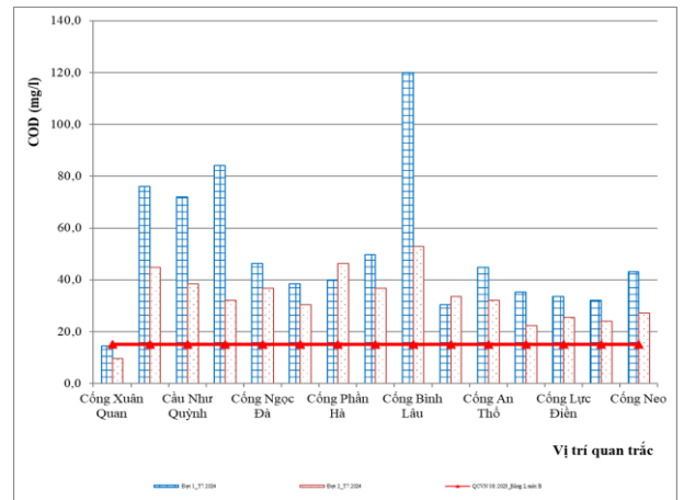
Hình 2.7. Diễn biến hàm lượng COD các đợt quan trắc trong tháng 7/2024
