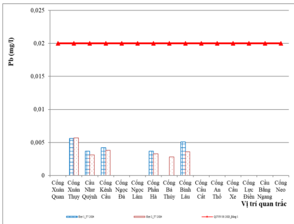
Hình 2.11. Diễn biến hàm lượng Pb các đợt quan trắc trong tháng 7/2024
