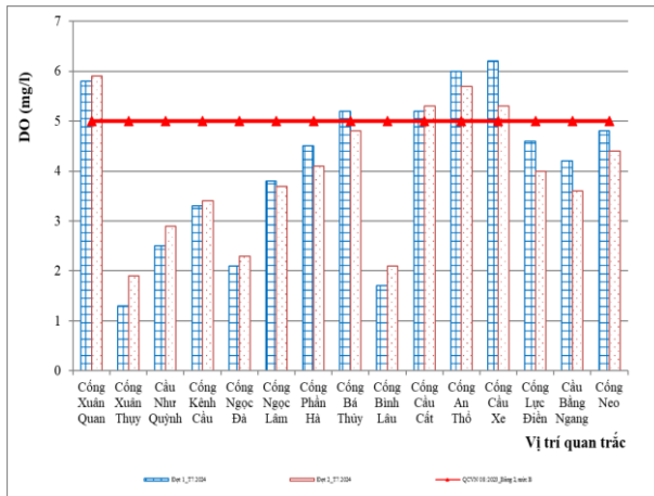
Hình 2.4. Diễn biến hàm lượng DO các đợt quan trắc trong tháng 7/2024
