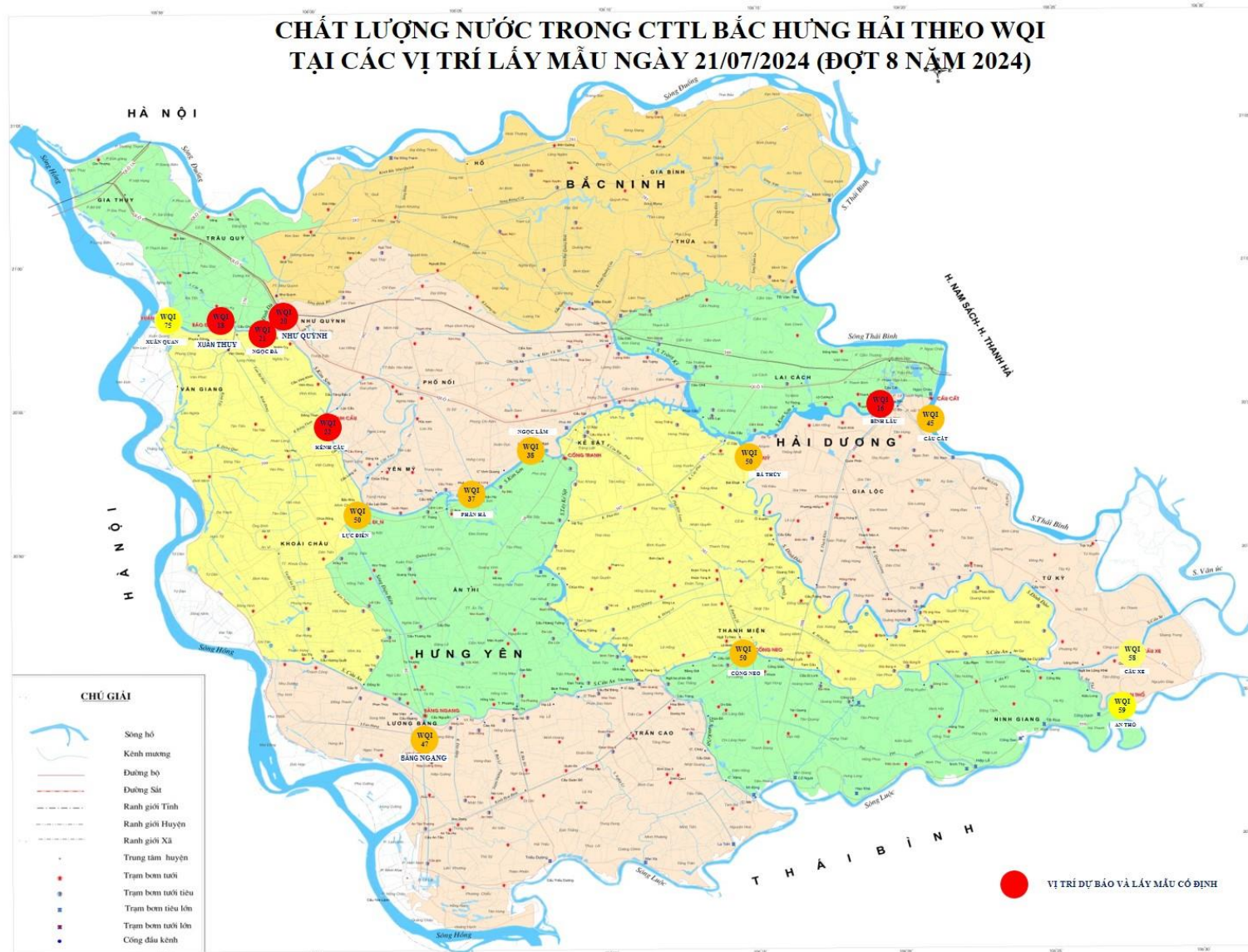
Hình 2.3. Chất lượng nước trong CTTL Bắc Hưng Hải theo chỉ số WQI tại các vị trí lấy mẫu ngày 21/07/2024 (đợt 2_tháng 7/2024)
