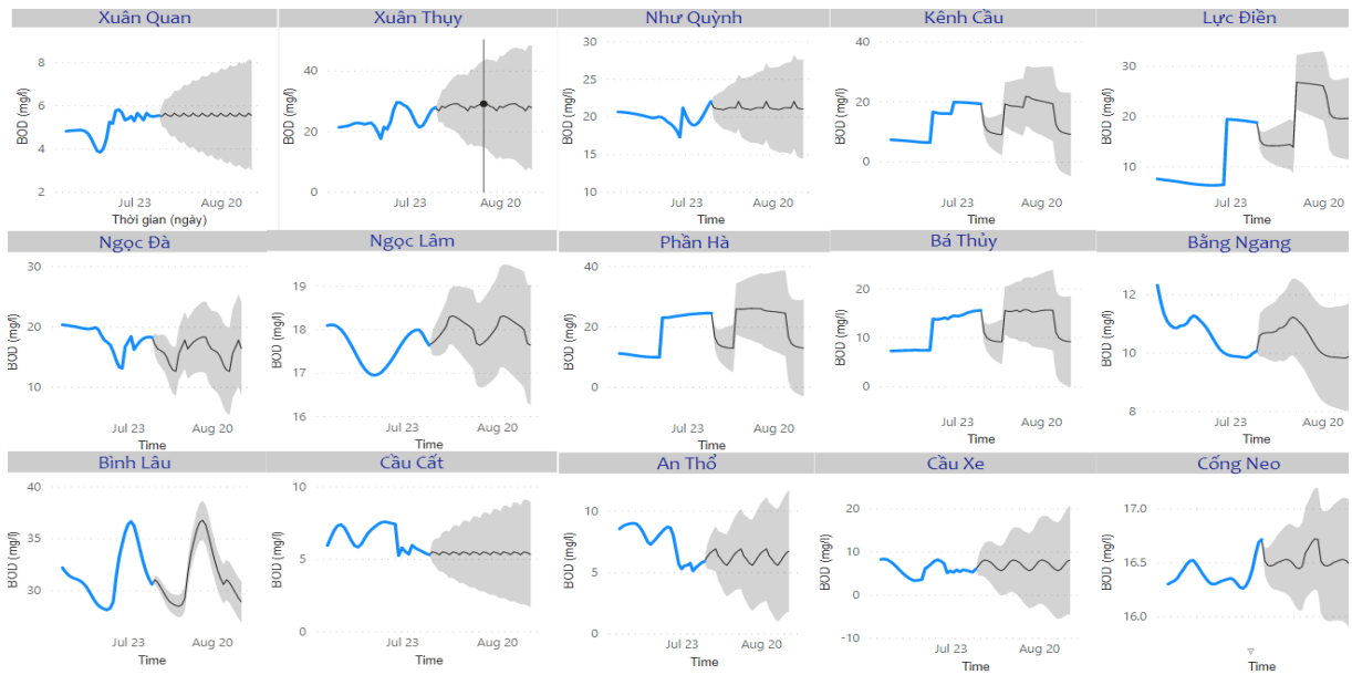
Hình 1.4. Biểu đồ dự báo BOD 5 hệ thống BHH (tháng 8/2024)
