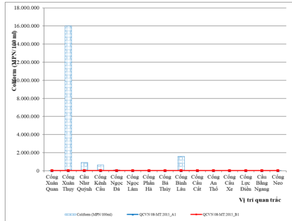
Hình 2.8. Diễn biến hàm lượng Coliform đợt quan trắc ngày 9/8/2022
