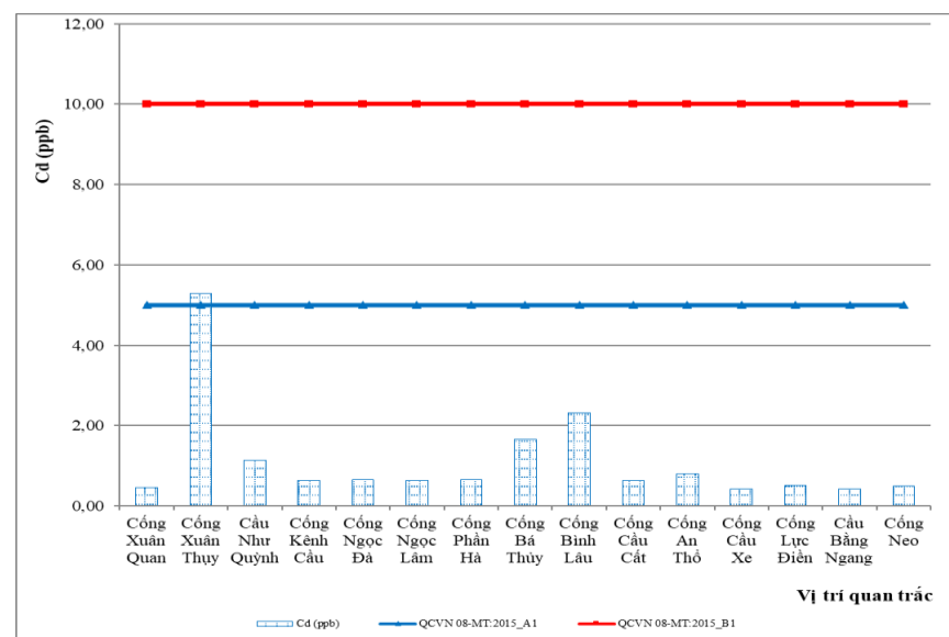
Hình 2.11. Diễn biến hàm lượng Cd đợt quan trắc ngày 9/8/2022
