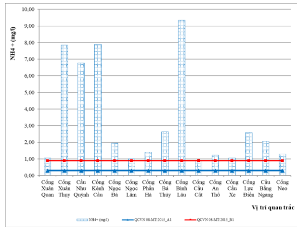
Hình 2.5. Diễn biến hàm lượng NH 4 + đợt quan trắc ngày 9/8/2022
