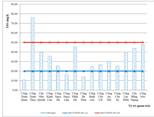
Hình 2.2. Diễn biến hàm lượng TSS đợt quan trắc ngày 9/8/2022
