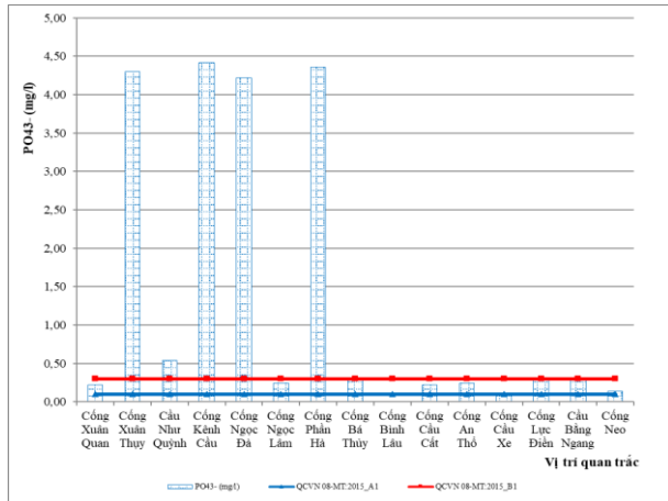
Hình 2.7. Diễn biến hàm lượng PO_4^{3-} đợt quan trắc ngày 9/8/2022
