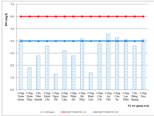
Hình 2.1. Diễn biến hàm lượng DO đợt quan trắc ngày 9/8/2022
