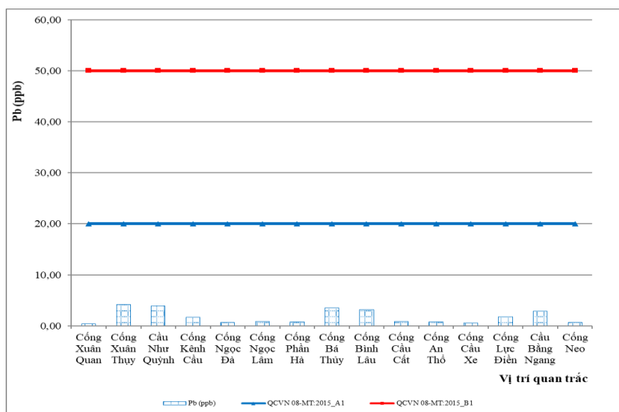
Hình 2.10. Diễn biến hàm lượng Pb đợt quan trắc ngày 9/8/2022
