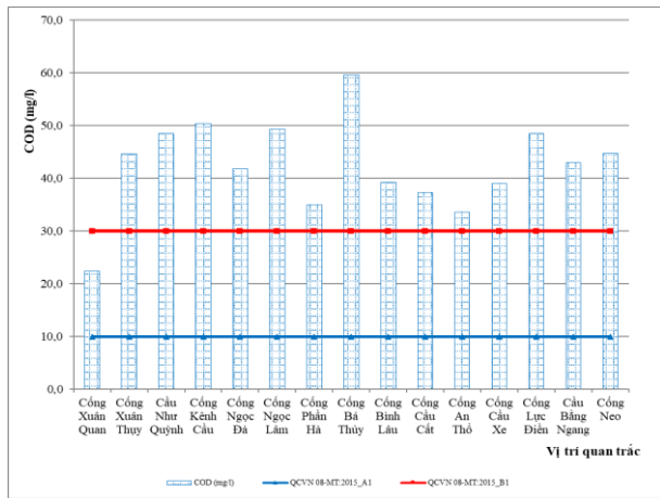
Hình 2.4. Diễn biến hàm lượng COD đợt quan trắc ngày 9/8/2022
