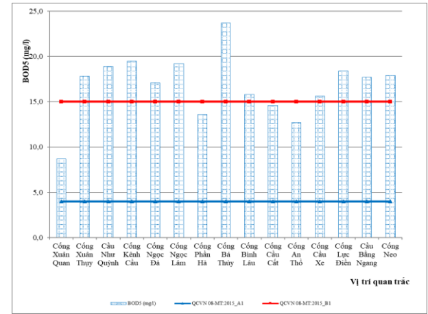
Hình 2.3. Diễn biến hàm lượng BOD 5 đợt quan trắc ngày 9/8/2022
