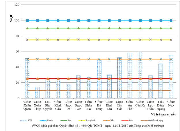
Hình 2.9. Diễn biến chỉ số WQI đợt quan trắc ngày 9/8/2022
