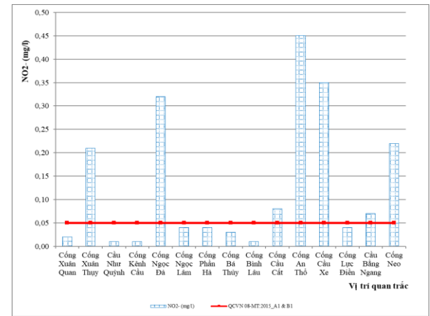
Hình 2.6. Diễn biến hàm lượng NO 2 - đợt quan trắc ngày 9/8/2022
