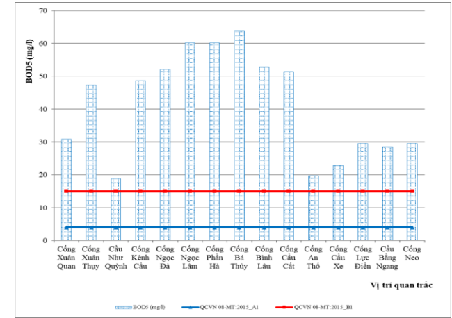
Hình 2.3. Diễn biến hàm lượng BOD 5 đợt quan trắc ngày 21/2/2022
