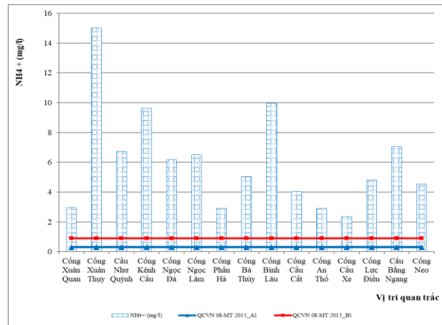
Hình 2.5. Diễn biến hàm lượng NH 4 + đợt quan trắc ngày 21/2/2022
