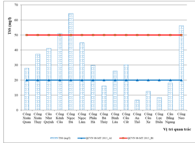
Hình 2.2. Diễn biến hàm lượng TSS đợt quan trắc ngày 21/2/2022
