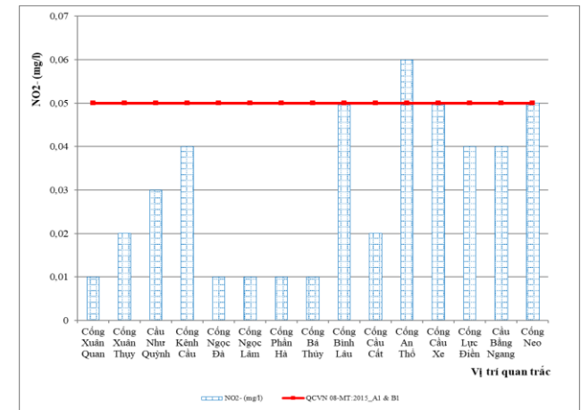
Hình 2.6. Diễn biến hàm lượng NO 2 - đợt quan trắc ngày 21/2/2022
