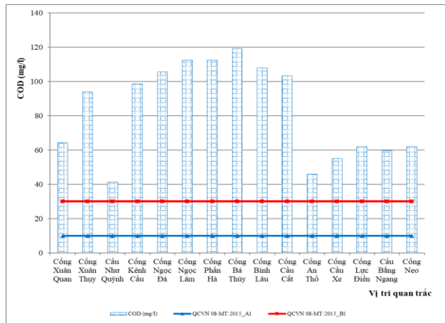
Hình 2.4. Diễn biến hàm lượng COD đợt quan trắc ngày 21/2/2022
