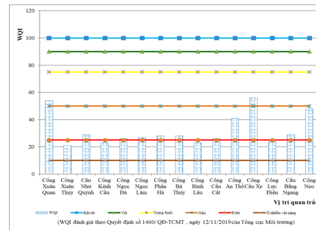
Hình 2.9. Diễn biến chỉ số WQI đợt quan trắc ngày 21/2/2022
