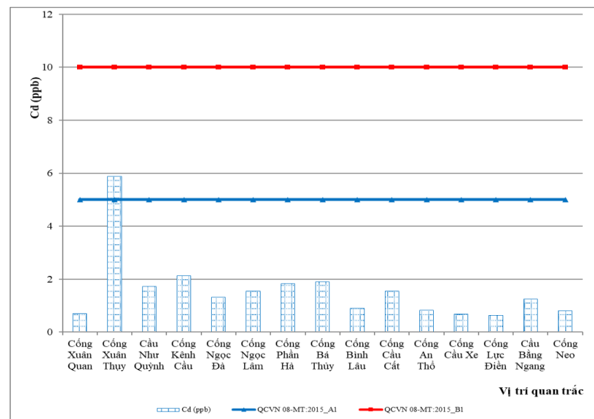
Hình 2.11. Diễn biến hàm lượng Cd đợt quan trắc ngày 21/2/2022
