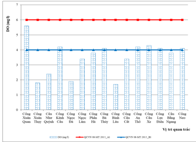
Hình 2.1. Diễn biến hàm lượng DO đợt quan trắc ngày 21/2/2022
