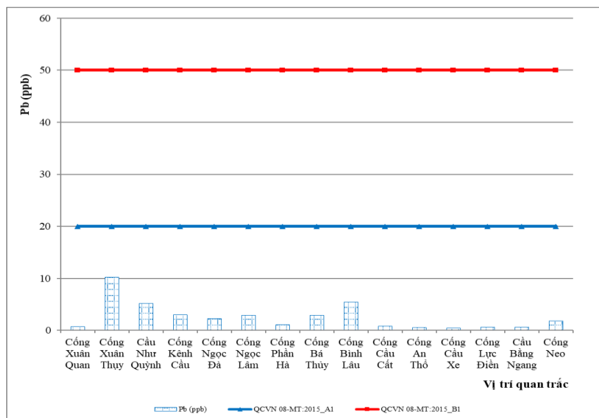
Hình 2.10. Diễn biến hàm lượng Pb đợt quan trắc ngày 21/2/2022
