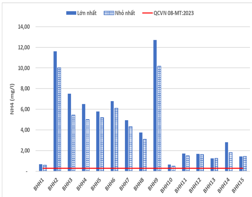
Biểu đồ dự báo NH 4 +
