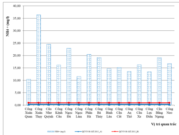
Hình 2.5. Diễn biến hàm lượng NH4+ đợt quan trắc ngày 22/7/2023
