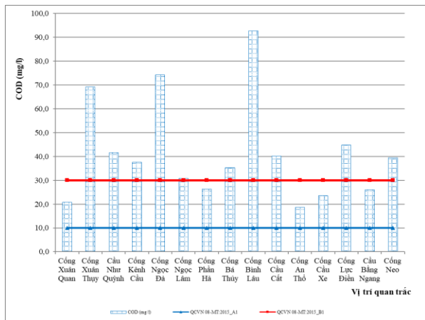
Hình 2.4. Diễn biến hàm lượng COD đợt quan trắc ngày 22/7/2023
