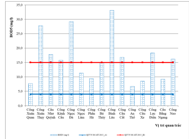
Hình 2.3. Diễn biến hàm lượng BOD5 đợt quan trắc ngày 22/7/2023
