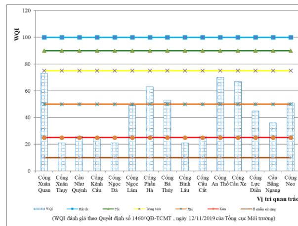
Hình 2.9. Diễn biến chỉ số WQI đợt quan trắc ngày 22/7/2023
