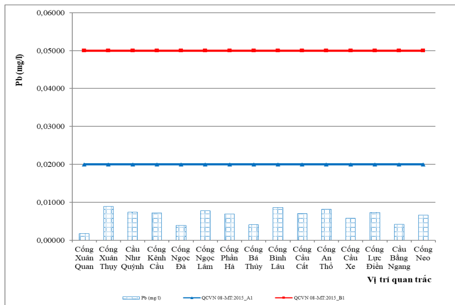
Hình 2.10. Diễn biến hàm lượng Pb đợt quan trắc ngày 22/7/2023
