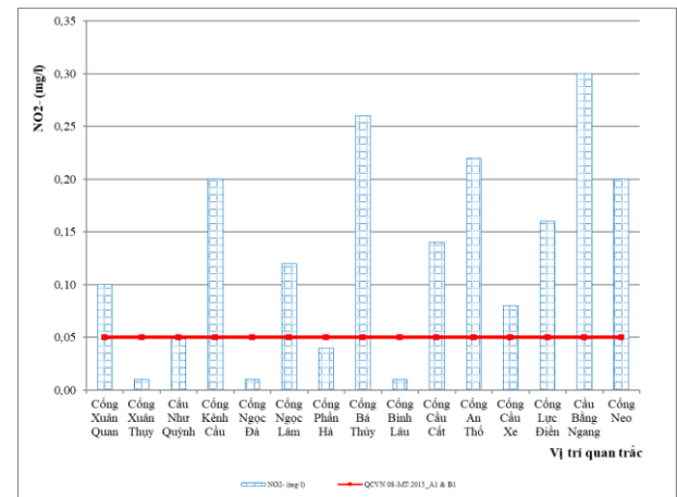
Hình 2.6. Diễn biến hàm lượng NO2- đợt quan trắc ngày 22/7/2023
