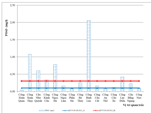
Hình 2.7. Diễn biến hàm lượng PO_4^{3-} đợt quan trắc ngày 22/7/2023
