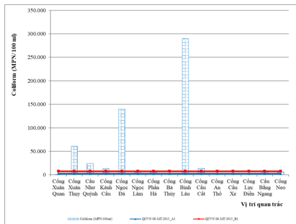
Hình 2.8. Diễn biến hàm lượng Coliform đợt quan trắc ngày 22/7/2023
