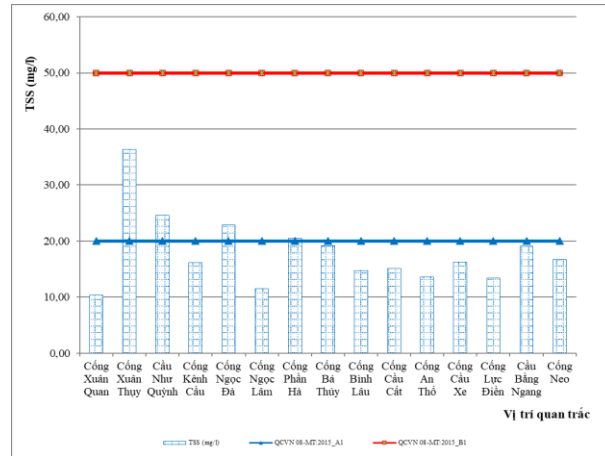
Hình 2.2. Diễn biến hàm lượng TSS đợt quan trắc ngày 22/7/2023
