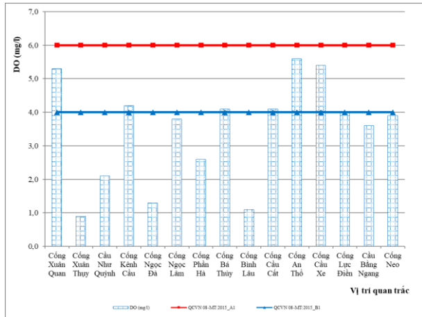
Hình 2.1. Diễn biến hàm lượng DO đợt quan trắc ngày 22/7/2023
