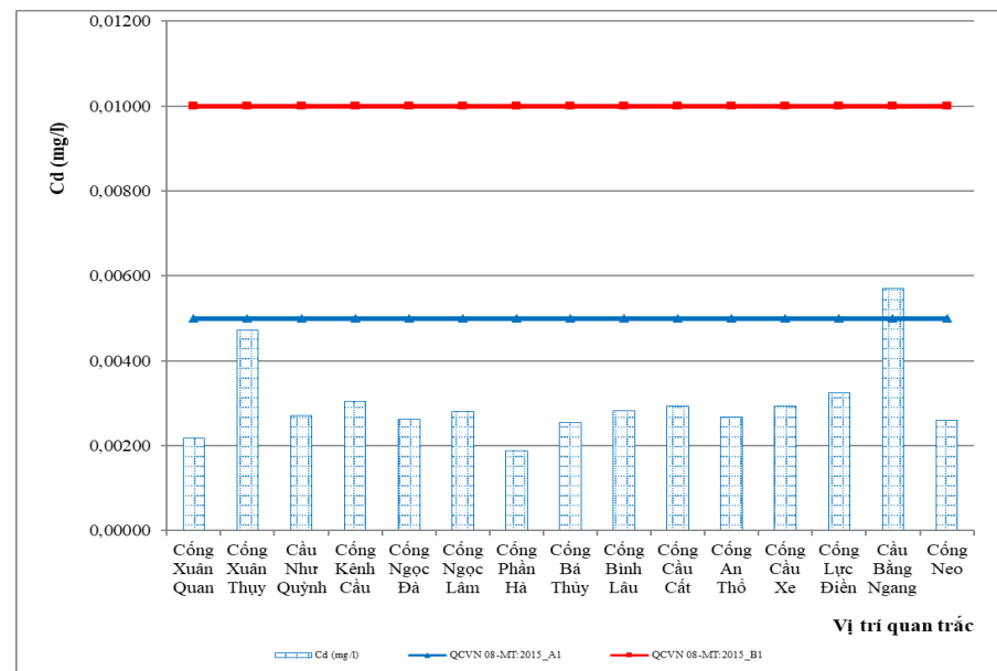
Hình 2.11. Diễn biến hàm lượng Cd đợt quan trắc ngày 22/7/2023
