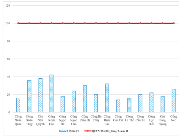
Hình 2. Diễn biến hàm lượng TSS đợt quan trắc ngày 3/7/2024
