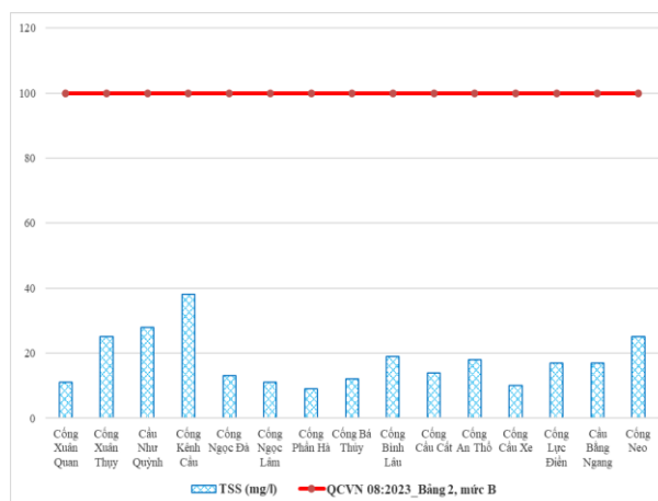
Hình 2. Diễn biến hàm lượng TSS đợt quan trắc ngày 15/2/2024
