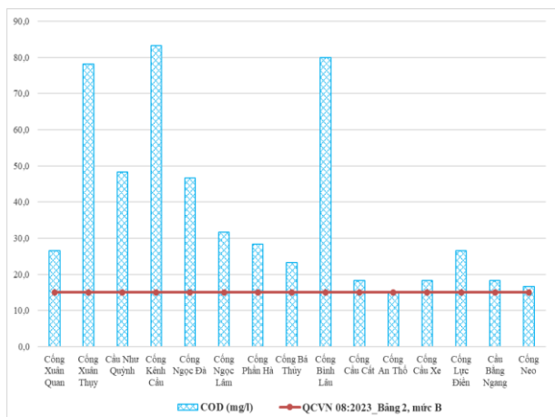
Hình 4. Diễn biến hàm lượng COD đợt quan trắc ngày 15/2/2024
