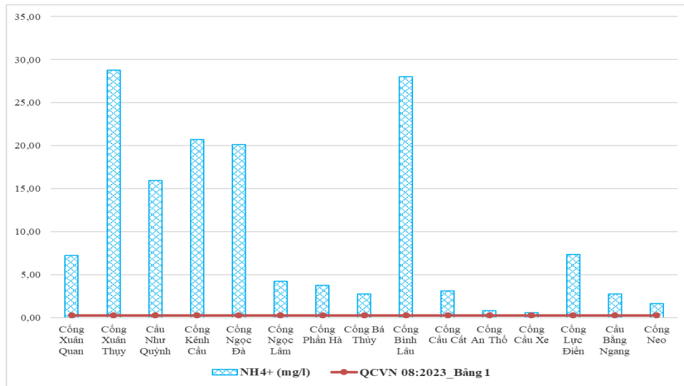
Hình 7. Diễn biến hàm lượng NH 4 + đợt quan trắc ngày 15/2/2024
