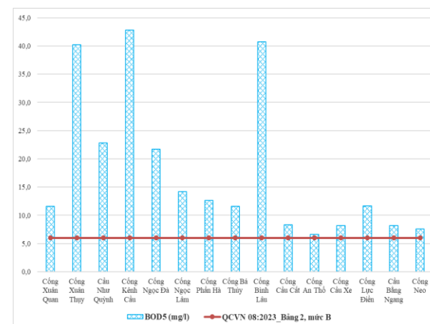
Hình 3. Diễn biến hàm lượng BOD 5 đợt quan trắc ngày 15/2/2024
