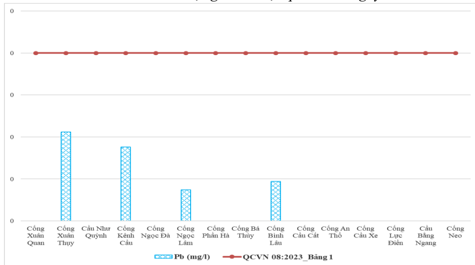
Hình 9. Diễn biến hàm lượng Pb đợt quan trắc ngày 15/2/2024
