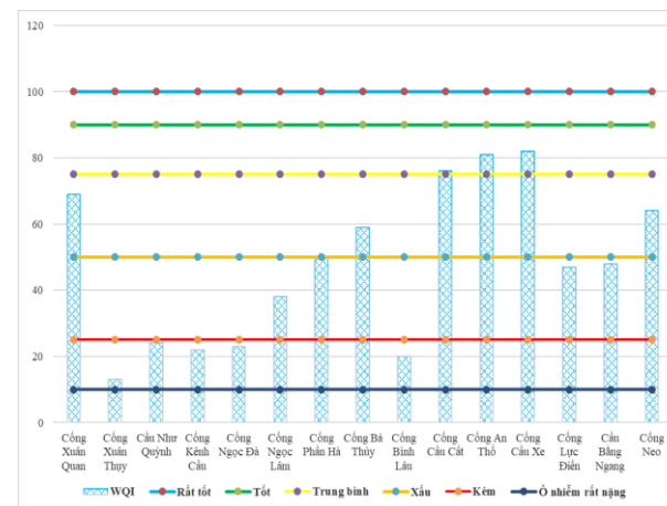
Hình 6. Diễn biến chỉ số WQI đợt quan trắc ngày 15/2/2024
