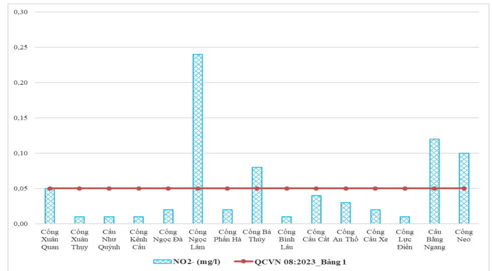
Hình 8. Diễn biến hàm lượng NO 2 - đợt quan trắc ngày 15/2/2024
