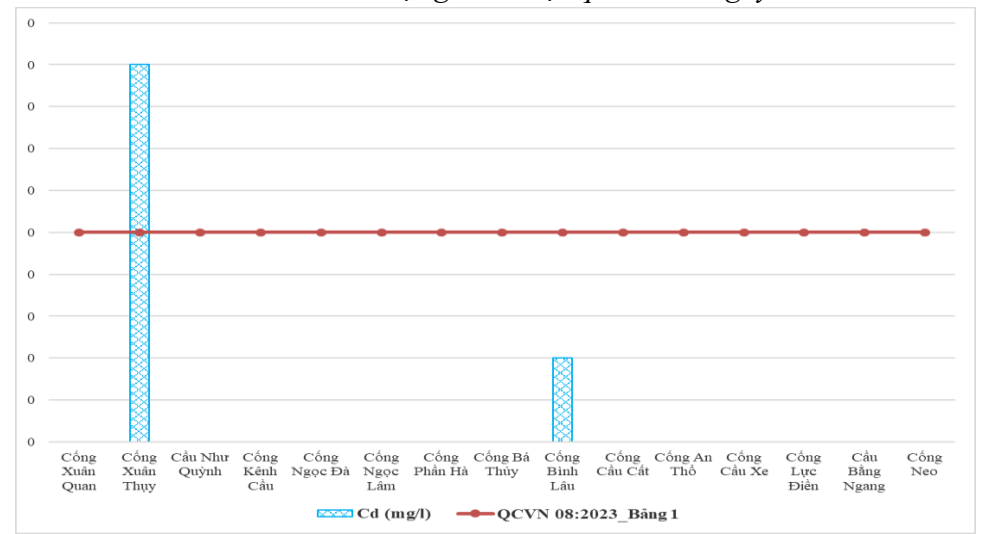
Hình 10. Diễn biến hàm lượng Cd đợt quan trắc ngày 15/2/2024
