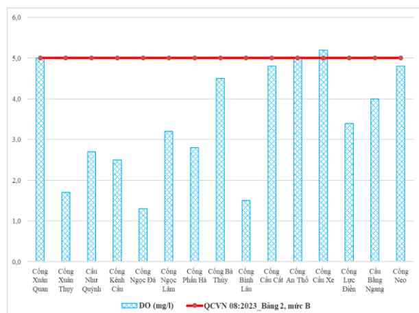
Hình 1. Diễn biến hàm lượng DO đợt quan trắc ngày 15/2/2024
