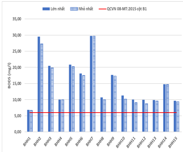
Biểu đồ dự báo BOD 5
