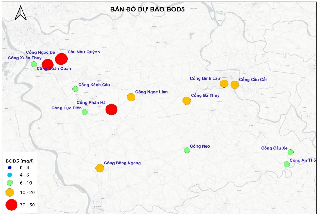
Bản đồ dự báo BOD 5 (Đợt 1)
