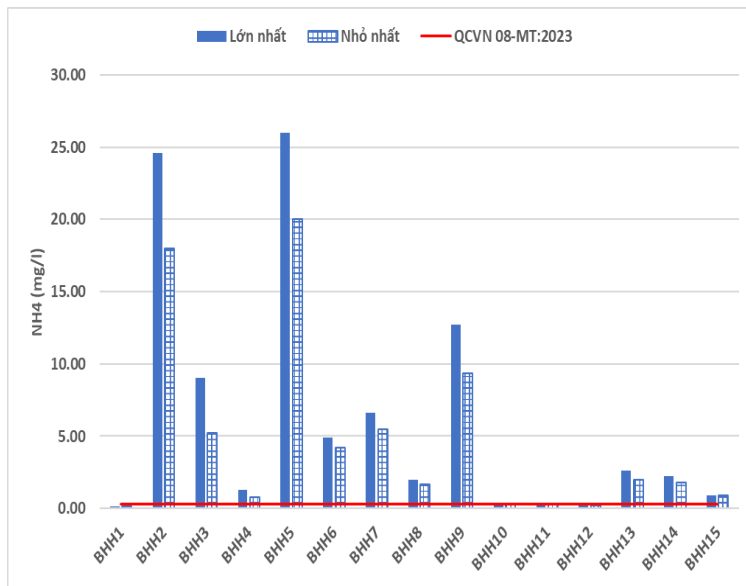
Biểu đồ dự báo NH 4 +
