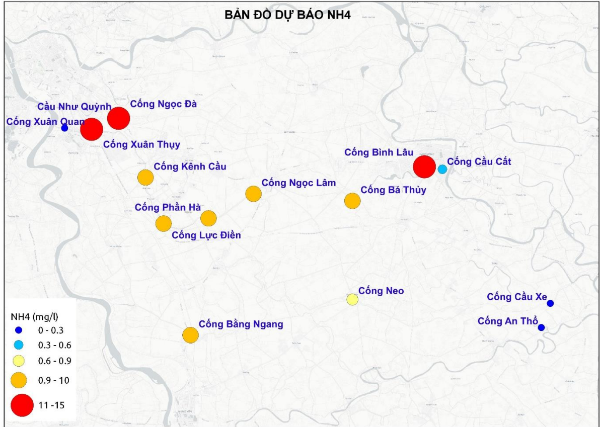
Bản đồ dự báo NH_4^+ (Đợt 1)
