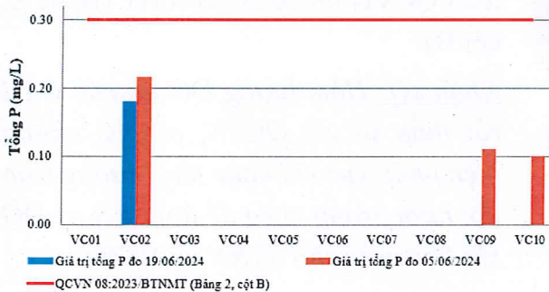
Hình 8: Biểu đồ giá trị Tổng P tại các vị trí lấy mẫu ngày 19/06/2024
