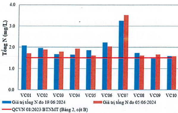
Hình 7: Biểu đồ giá trị Tổng N tại các vị trí lấy mẫu ngày 19/06/2024
