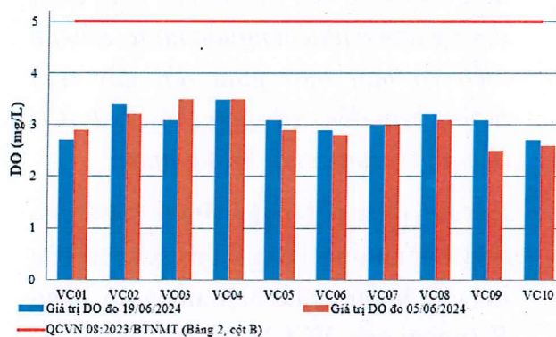
Hình 5: Biểu đồ giá trị DO tại các vị trí lấy mẫu ngày 19/06/2024
