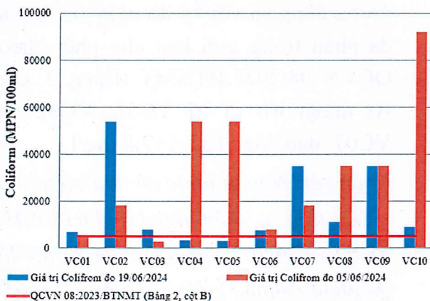
Hình 9: Biểu đồ giá trị Coliform tại các vị trí lấy mẫu ngày 19/06/2024
