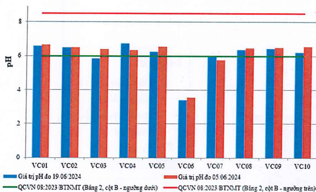
Hình 2: Biểu đồ giá trị pH tại các vị trí lấy mẫu ngày 19/06/2024
