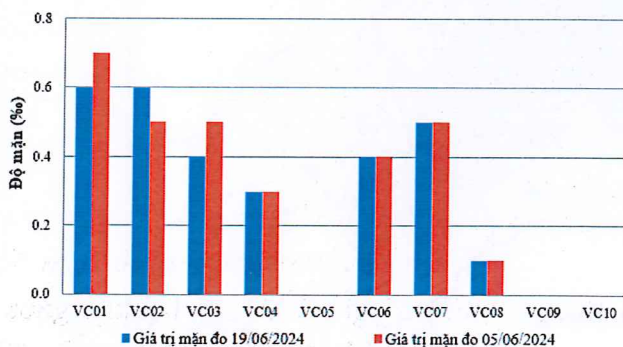
Hình 3: Biểu đồ giá trị mặn tại các vị trí lấy mẫu ngày 19/06/2024
