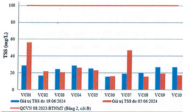
Hình 4: Biểu đồ giá trị TSS tại các vị trí lấy mẫu ngày 19/06/2024
